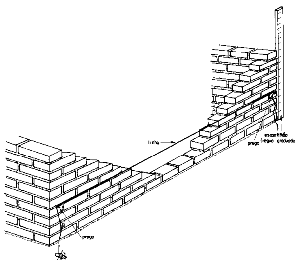
Detalhe do nivelamento da elevação da parede.
