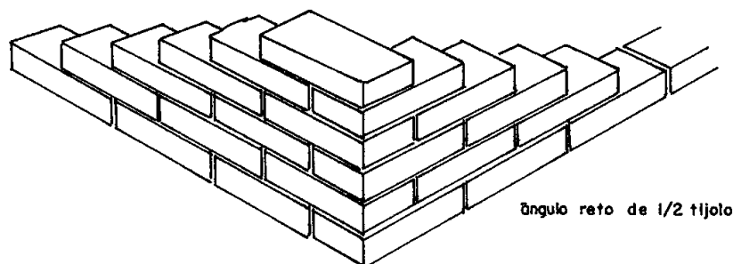
Canto em parede de meio tijolo no ajuste comum
